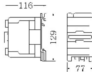
CJX2-40,50,63
