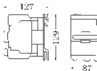
CJX2-80,95
